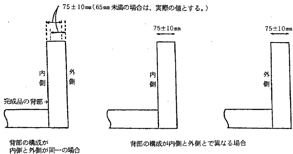
別図第 15 試験体の調整（背部の内側と外側の構成の差異）
