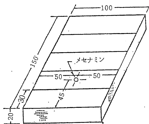
別図第10 火源の位置 (単位 mm)
