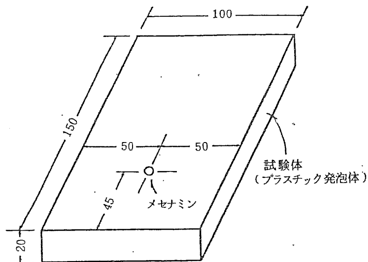
別図第11 火源の位置 (プラスチック発泡体) (単位 mm)
