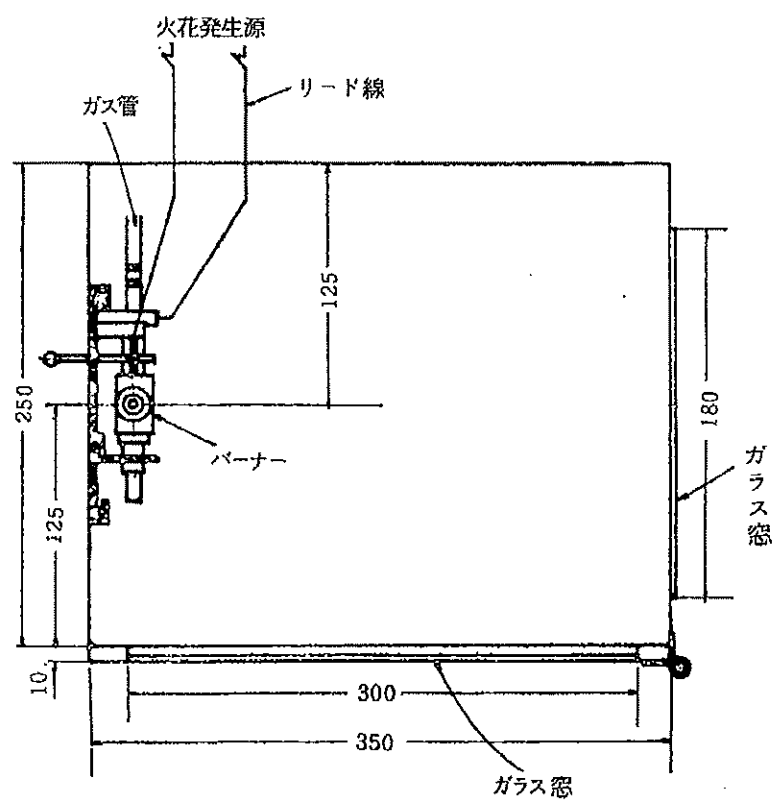
別図第19 電気火花発生装置
