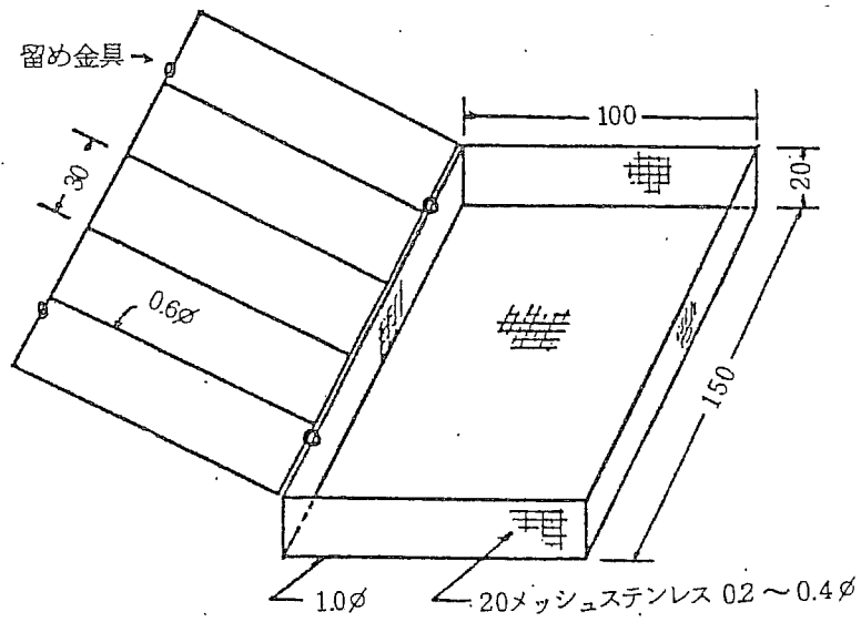
別図第9 バスケット (単位 mm)
