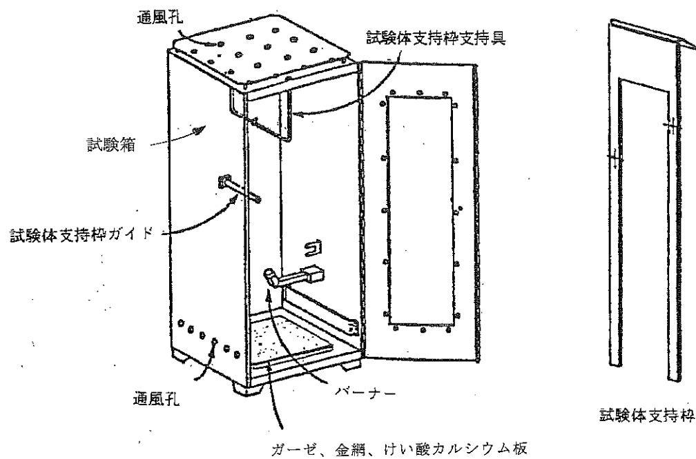
別図第 12 燃焼試験装置
