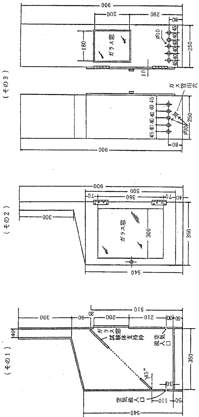
別図第1 燃焼試験箱 (単位 mm)
